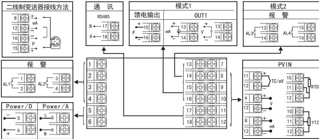
规格尺寸为H型接线图
