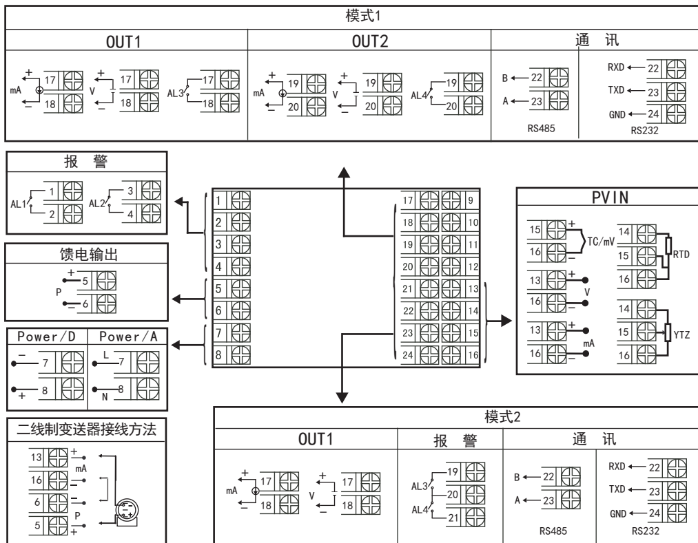
规格尺寸为F型接线图
